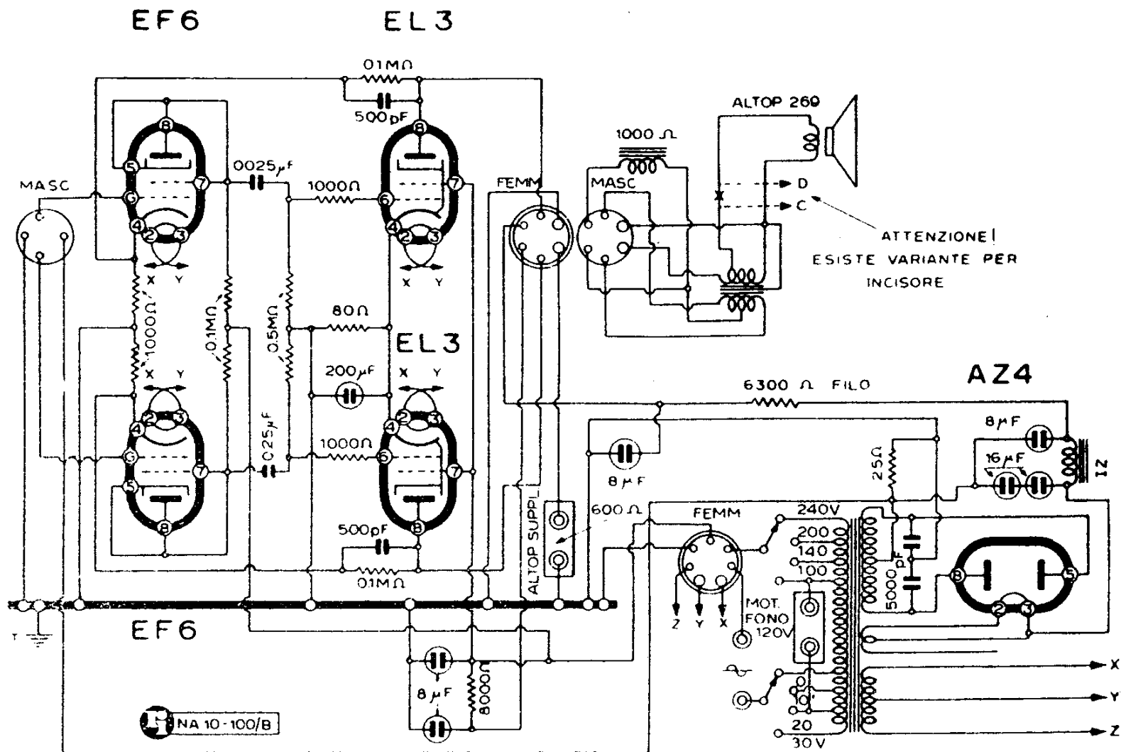
F.I.M.I. - MOD. PHONOLA « 902 » BE. - ALIM.
